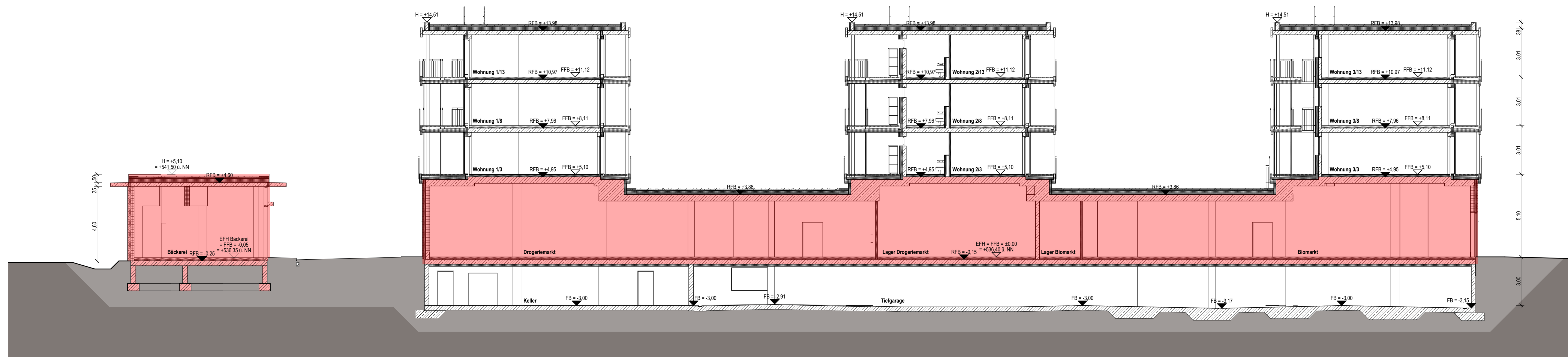
01 Schnitt A - A 1:100
