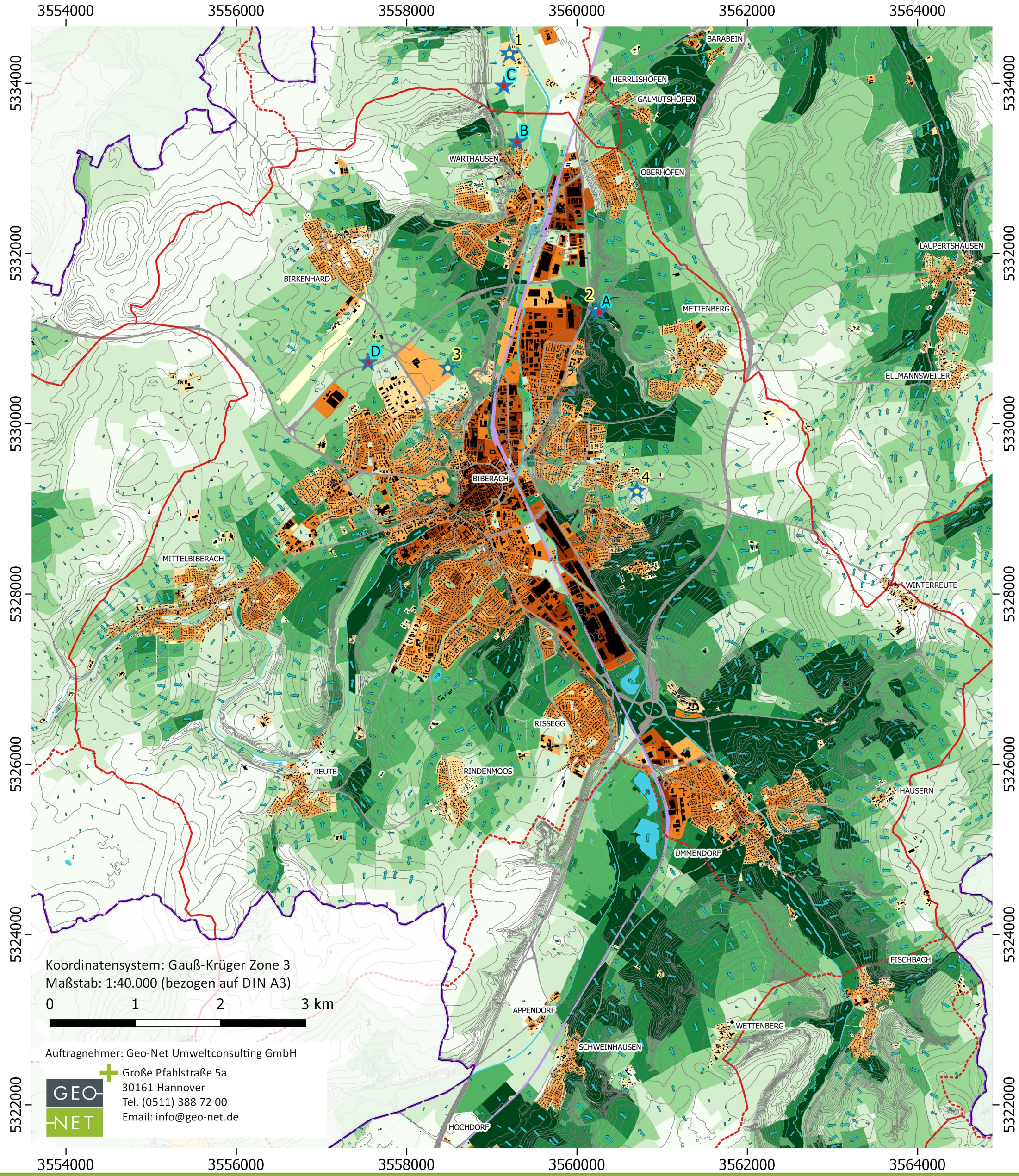
Klimaanalysekarte Verdichtungsraum Biberach
