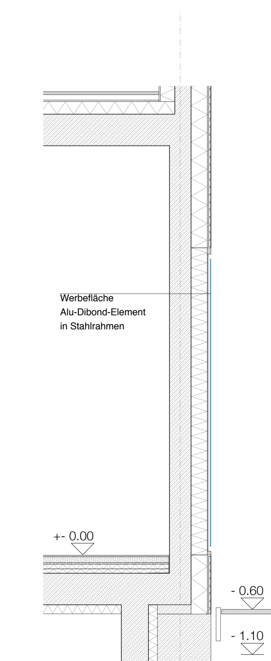
Werbefläche Schnitt M 1:25
