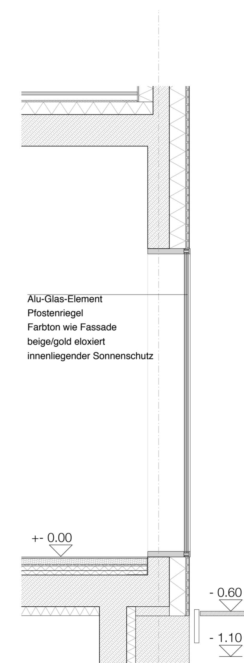
Backshop Schnitt M 1:25
