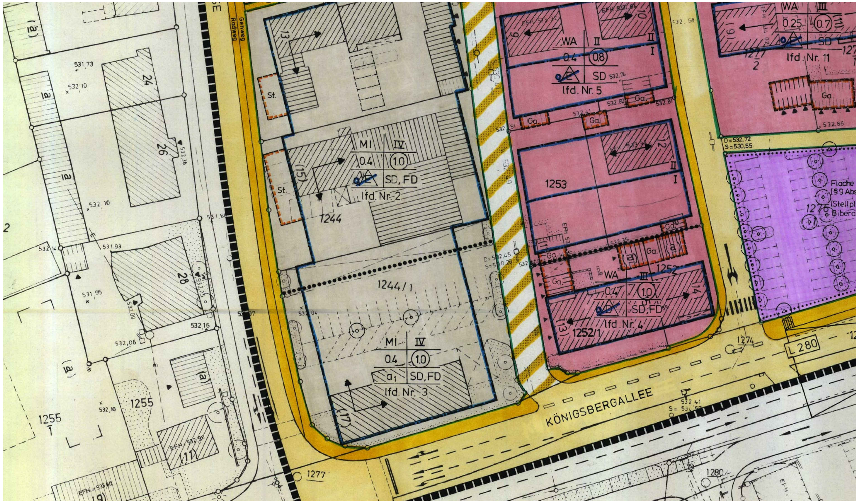
Auszug aus dem rechtskräftigen Bebauungsplan "Rollinstraße/Adenauerallee/Königsbergallee"
