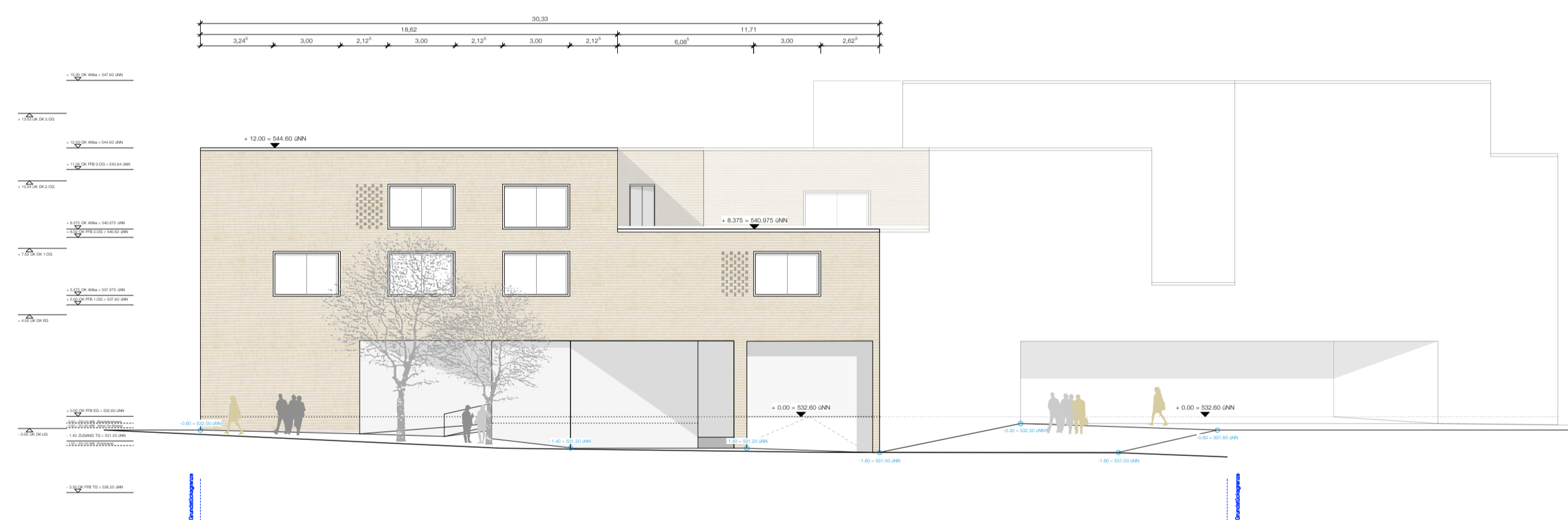
ANSICHT NORD
