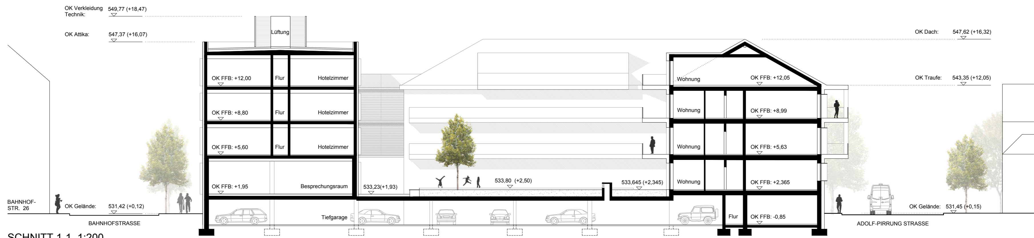
SCHNITT 1-1 1:200
