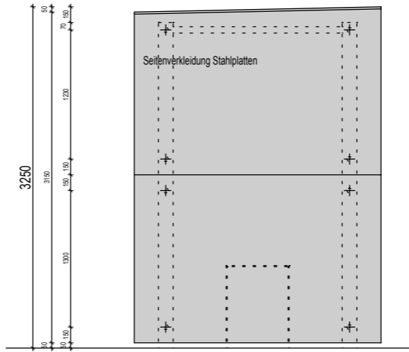
SCHNITT / ANSICHT
