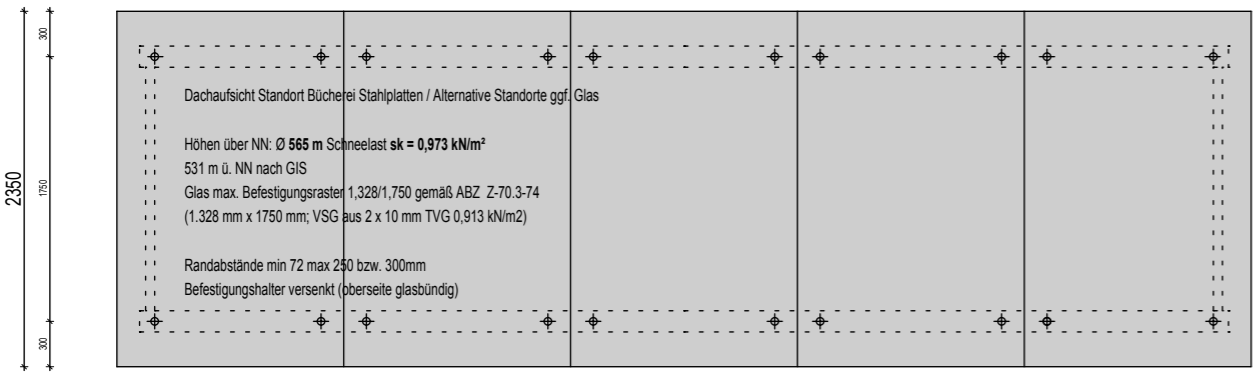
DACHAUFSICHT
