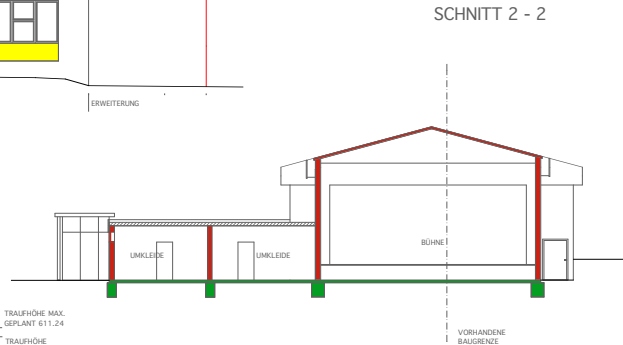
SCHNITT 2 - 2
