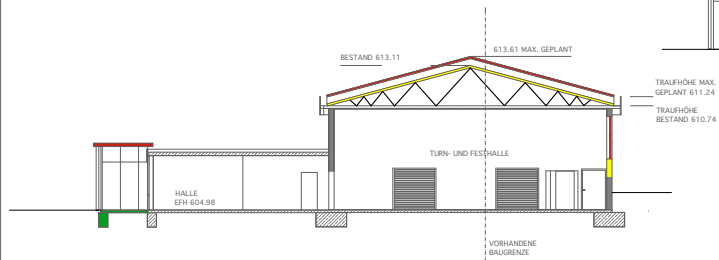
SCHNITT 1 - 1
