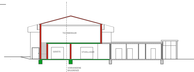
SCHNITT 3 - 3
