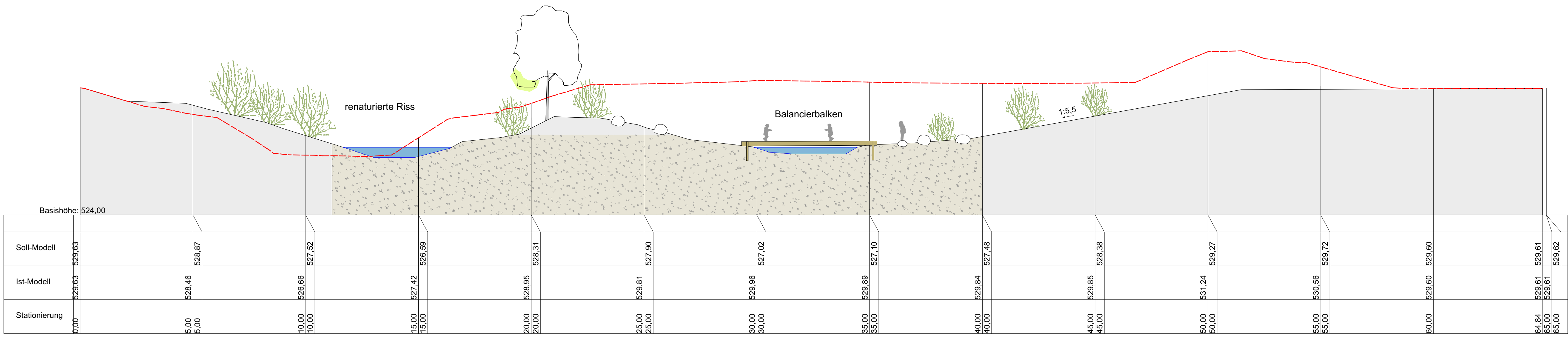
Schnitt A
