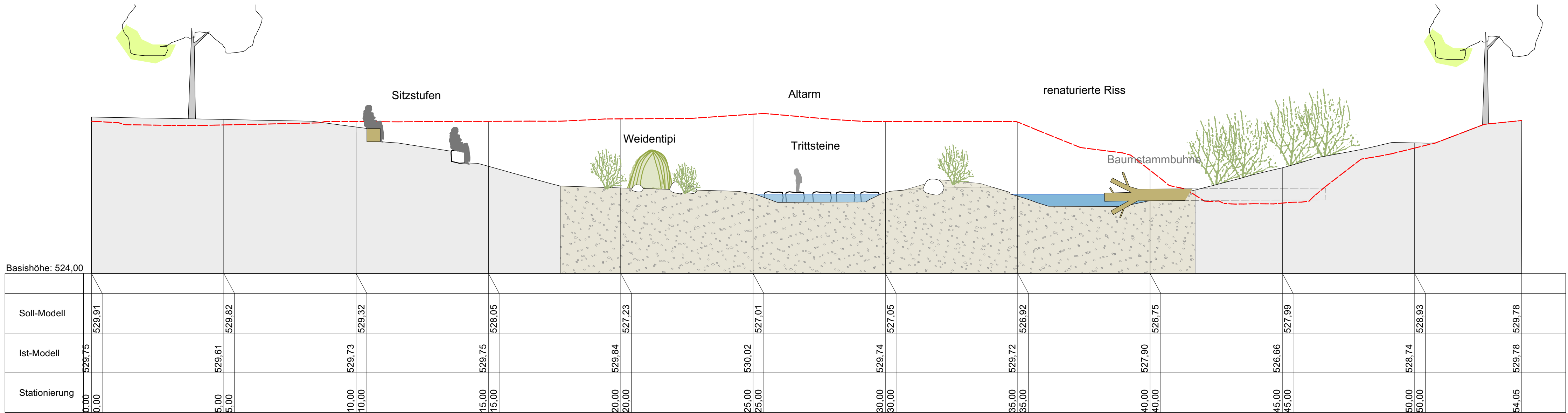
Schnitt B
